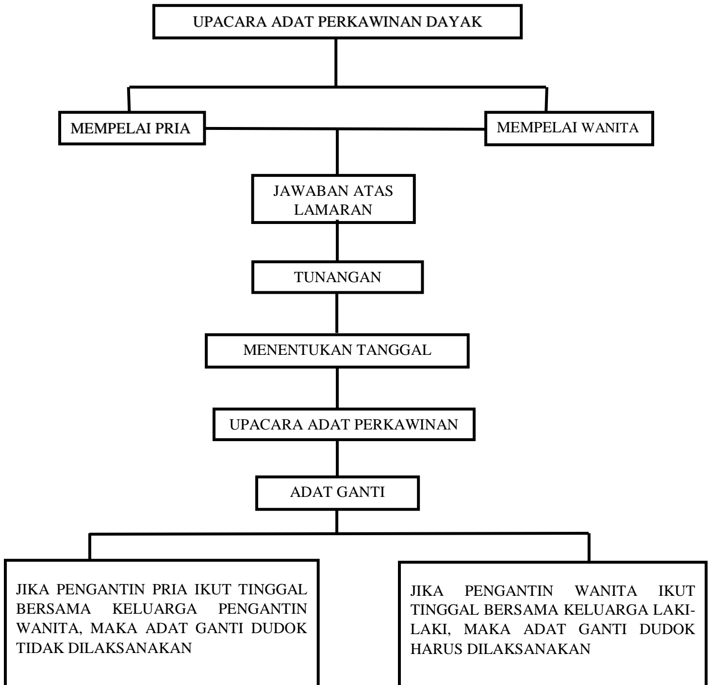
Gambar 1. 1 Kerangka Konsep
