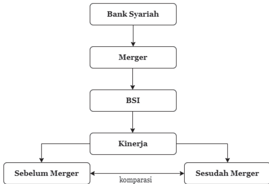
Gambar 2.1 Kerangka Konseptual
