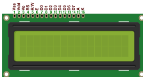
Gambar 2.6 Tampilan fisik LCD 16×2
