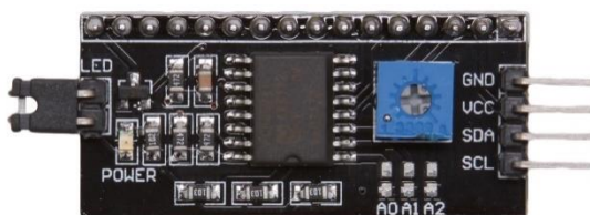
Gambar 2.7 Tampilan fisik modul I2C
