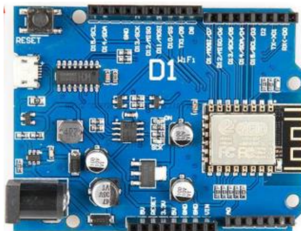
Gambar 2.8 Tampilan fisik WeMos D1 R2
